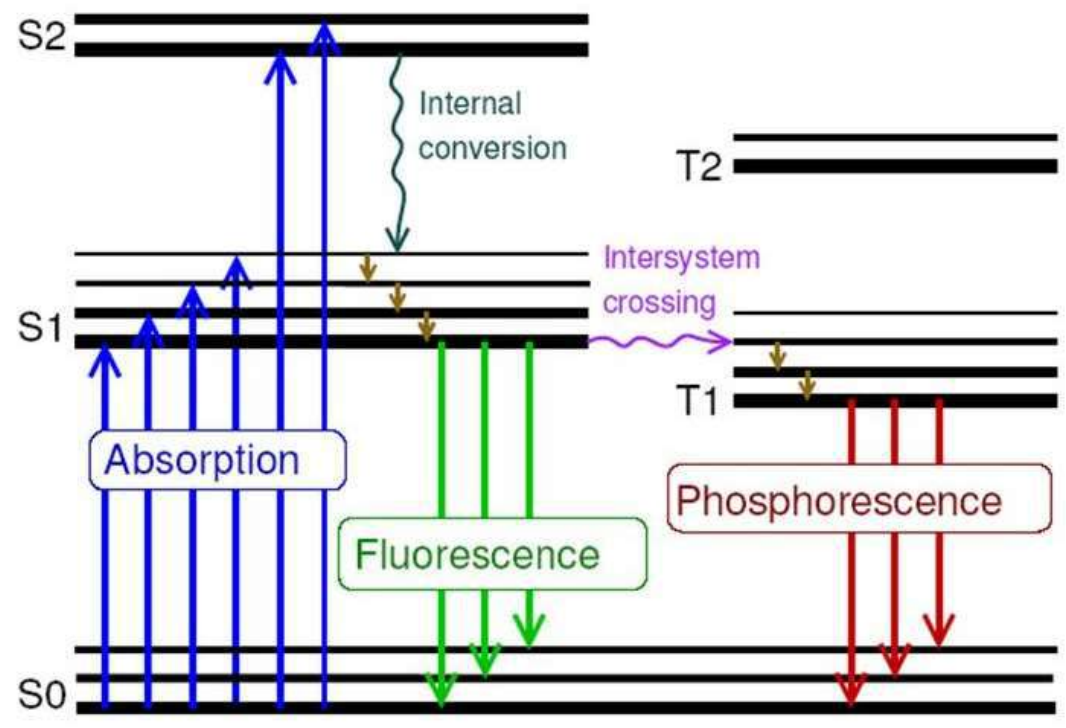
Jablonski diagram
